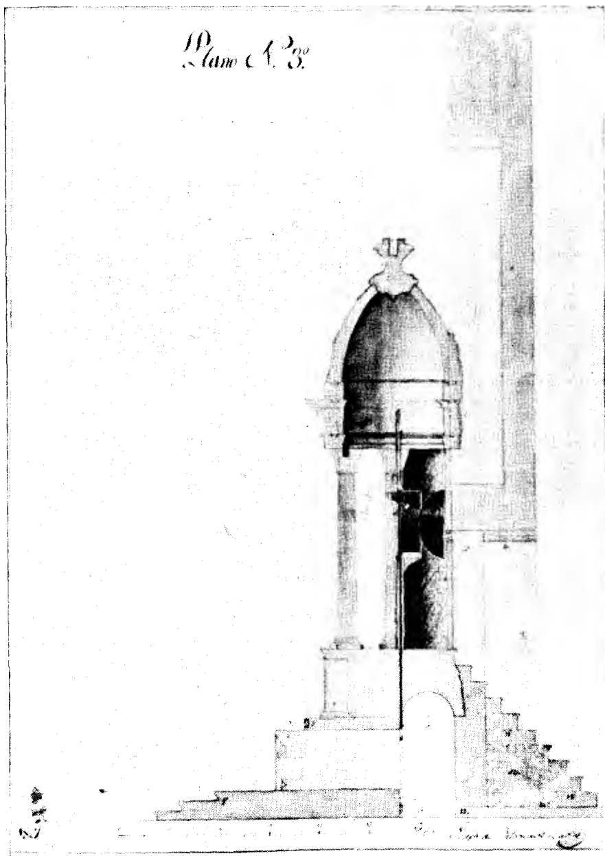
Fig. 4.- Sección perpendicular
